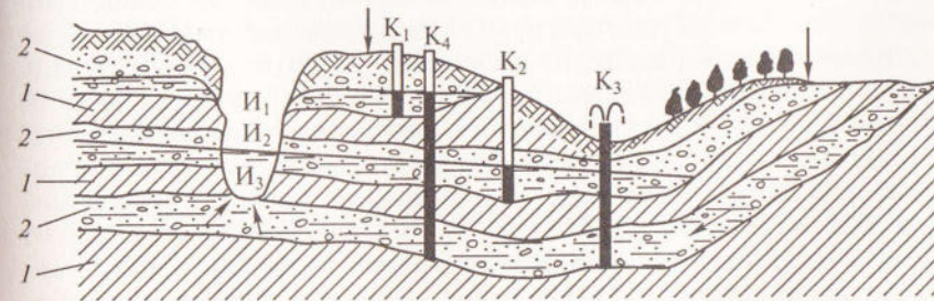
• Рис. 8.1. Схема образования и залегания подземных вод:
